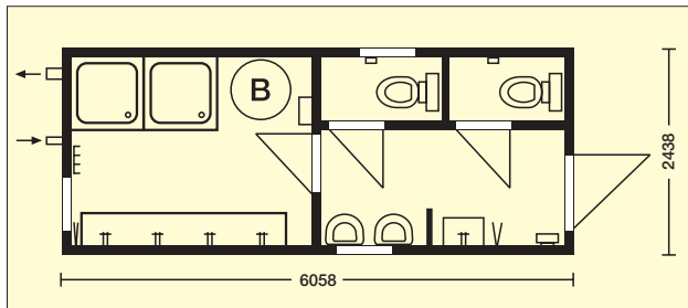
Beispiel einer Grundriss-/Ausstattungsvariante SC 20
